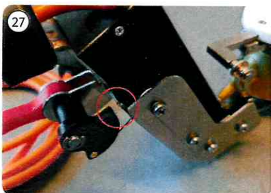
Finden Sie das Ende der Feder an der Unterseite des Gerätes in der Nähe des Metalldrahtes.
