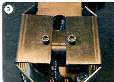
3 Lösen Sie die Schrauben auf der Unterseite des Hitzeschutzes.
