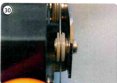
Überprüfen Sie, ob das Übertragungskabel richtig am Spannrad platziert ist.
