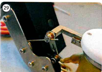
Setzen Sie die Feder wie hier abgebildet auf die Buchse.
